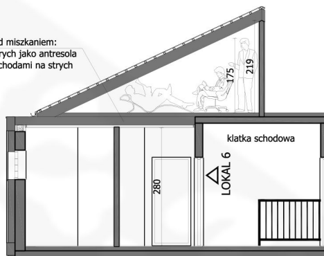
PRZEKRÓJ MIESZKANIA NR 6
