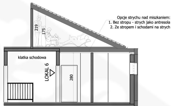
PRZĘKÓJ MIESZKANIA NR 6
