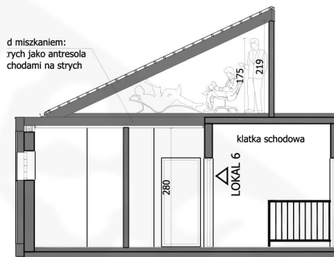
PRZEKRÓJ MIESZKANIA NR 6
