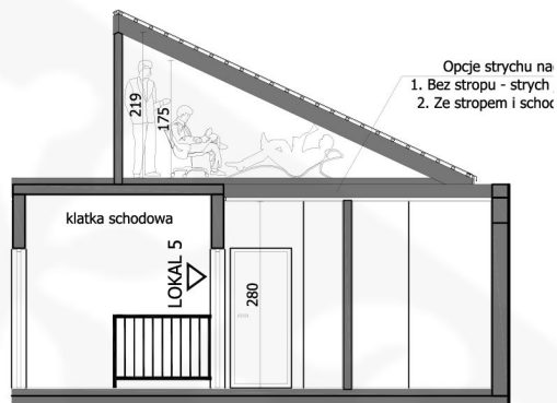
PRZEKRÓJ MIESZKANIA NR 5
